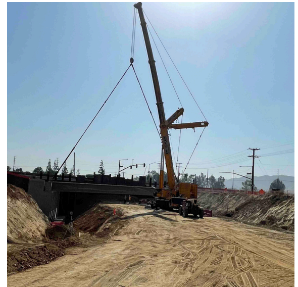
Mirando hacia el este en Jurupa Road hasta las etapas iniciales del nuevo puente Van Buren Boulevard, donde esta grúa colocó seis de las 12 vigas de hormigón de 17,000 libras de peso para el sistema de soporte del puente.
